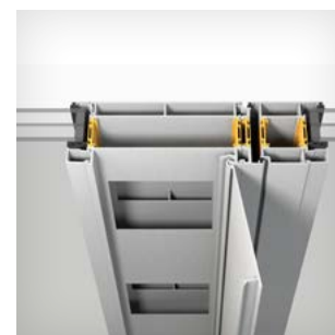
E-karm för Dörr 2086 Profil för elektronik.
