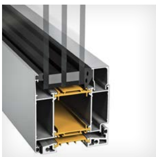
Dörr 2086 Extreme. Integrerad glasningslist.
