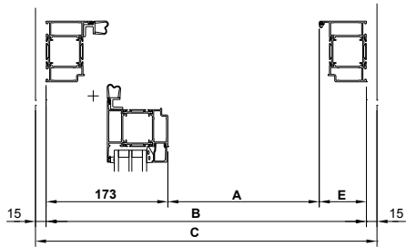
Dörr med klämfri bakkant med gummlist
