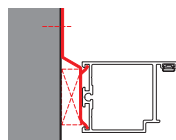
Karminfästning med vridankarjärn.
