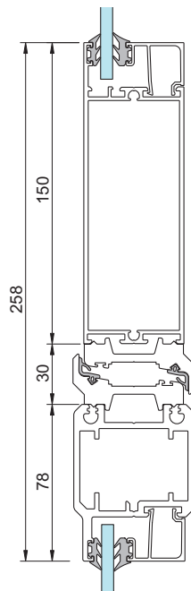
8 - Ö.K. dörr med överljus och profil för stor slagdörrsautomatik
