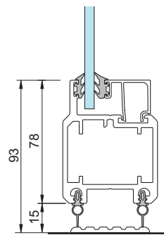
3 - Dörr med släptätning mot tröskel
